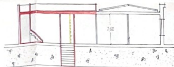
SECCION
